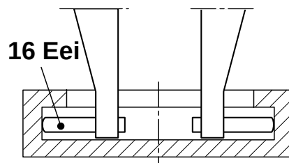
Mérőbetétek belső méréshez
