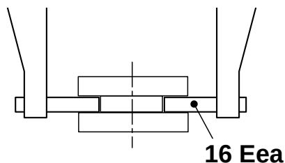
Mérőbetétek külső méréshez
